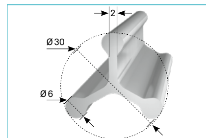
Wurstlattenprofil / Selchstab • Sausage Rack Bar
