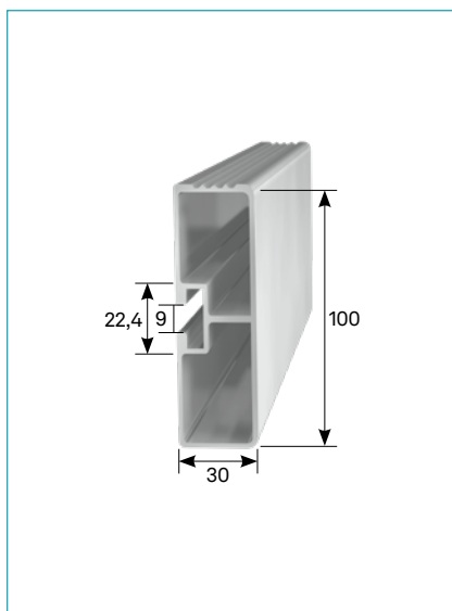
Unterfahrschutz • Cycle Protection Profile
