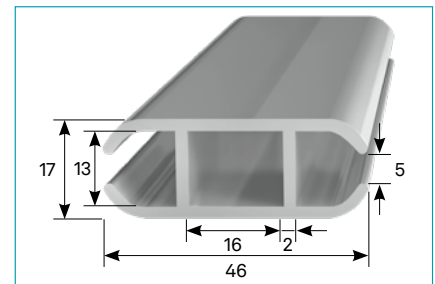
Kederleiste • Channel Rail
