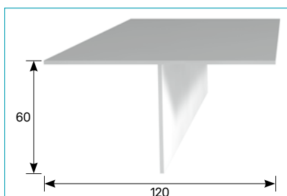
T-Profil • T-Profile
