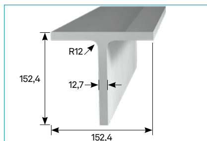
T-Profil mit Radius • T-Section with radius
