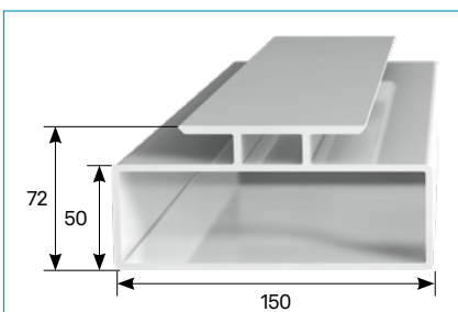
Bodenprofil • Floor Profile
