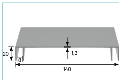
Leuchtkastenprofil • Light Box Profile
