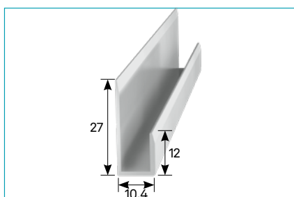
U-Profil ungleichschenkelig • U-Profile unequal
