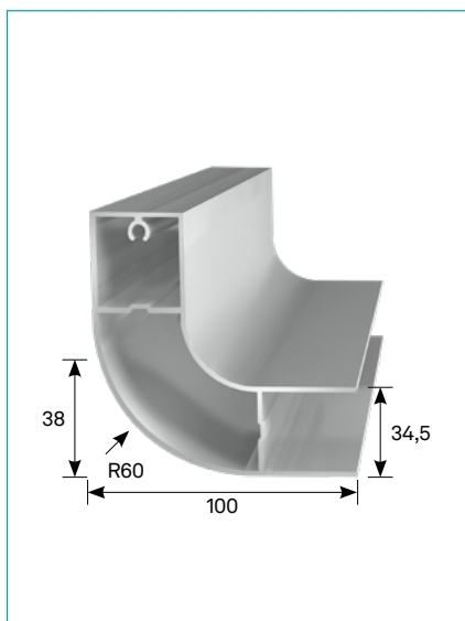
Abweiser • Rejection Profile
