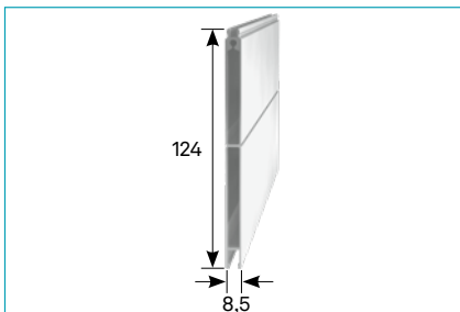
Sichtschutzprofil • Sight Protection Profile
