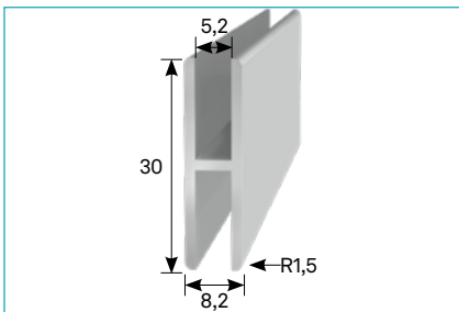
H-Profil • H-Section
