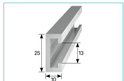
Abdeckleiste • Cover Strip
