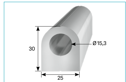
Scharnier- und Riegelprofil • Hinge and Bolt Profile
