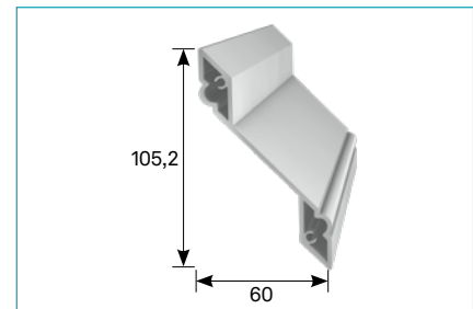
Dekor-Lamelle 45° • Decor-Slat 45°
