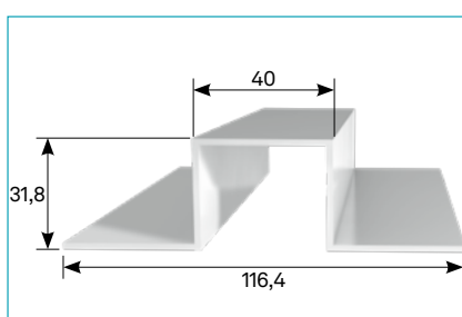
Omega-Profil • Omega Profile
