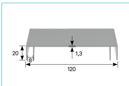
Leuchtkastenprofil • Light Box Profile
