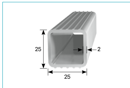
Leitersprosse • Rung
