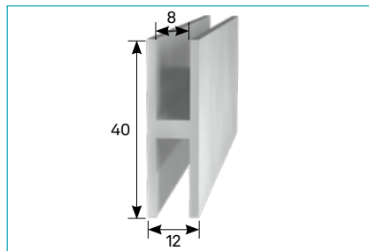
H-Profil • H-Section
