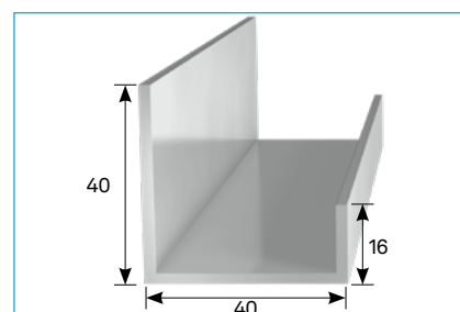
U-Profil ungleichschenkelig • U-Profile unequal
