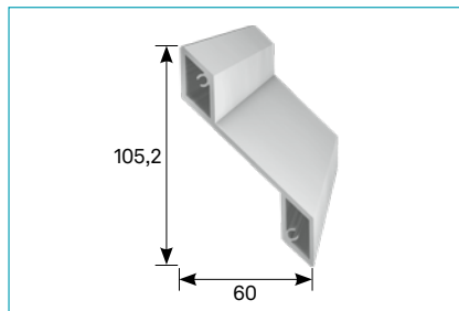
Lamelle 45° • Slat 45°
